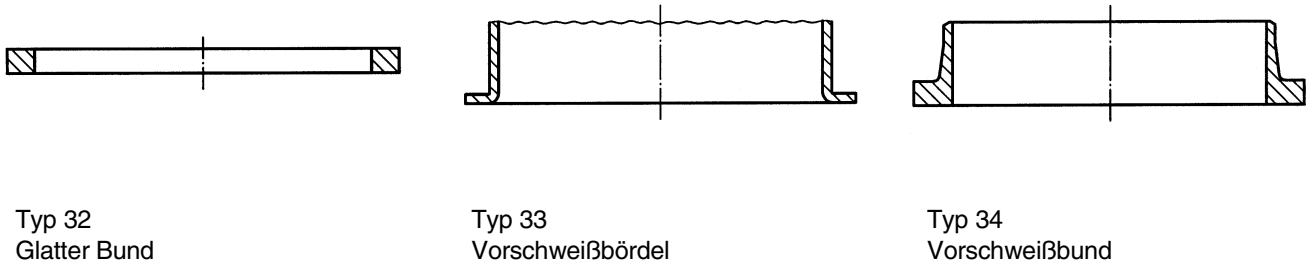
Bild 2 — Zugehörige Bauteile Typen 32 bis 34
